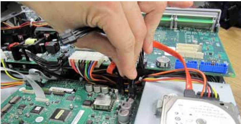
Figure 48: Attach Power cable to AMB
